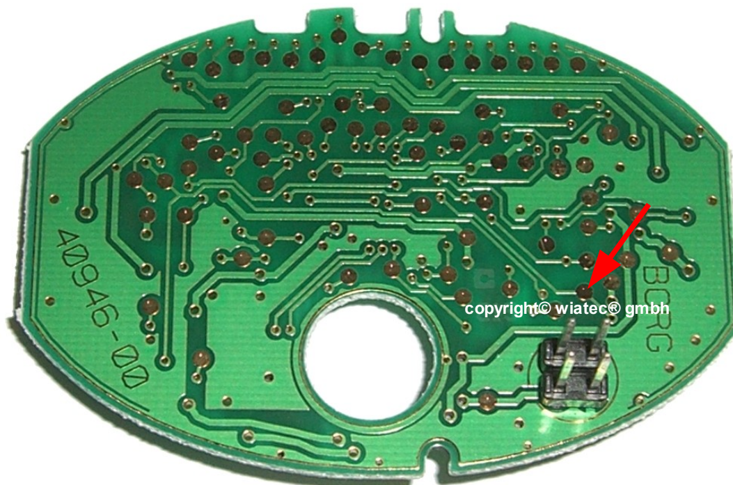
Abbildung 2: Anschlusspunkt (roter Pfeil) für die MG Steuerleitung (braun, nicht im Bild dargestellt)
